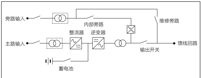
单机示意图
