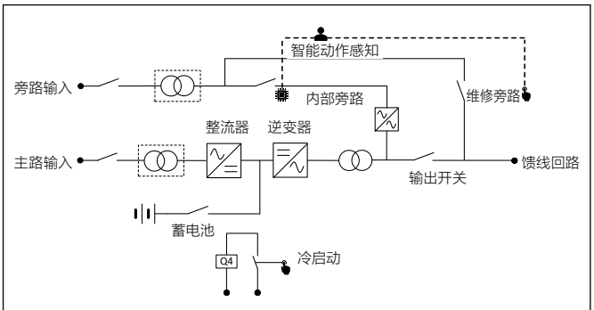
单机示意图
