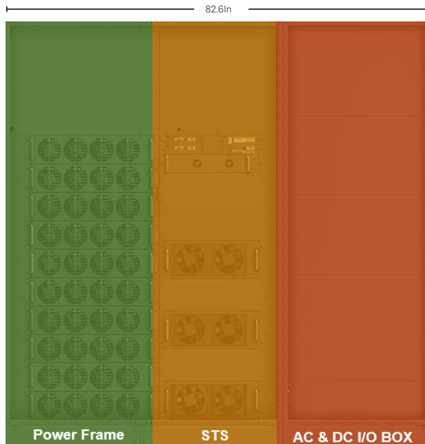
1.25MW 480Vac 3W Vertiv™ PowerUPS 9000
