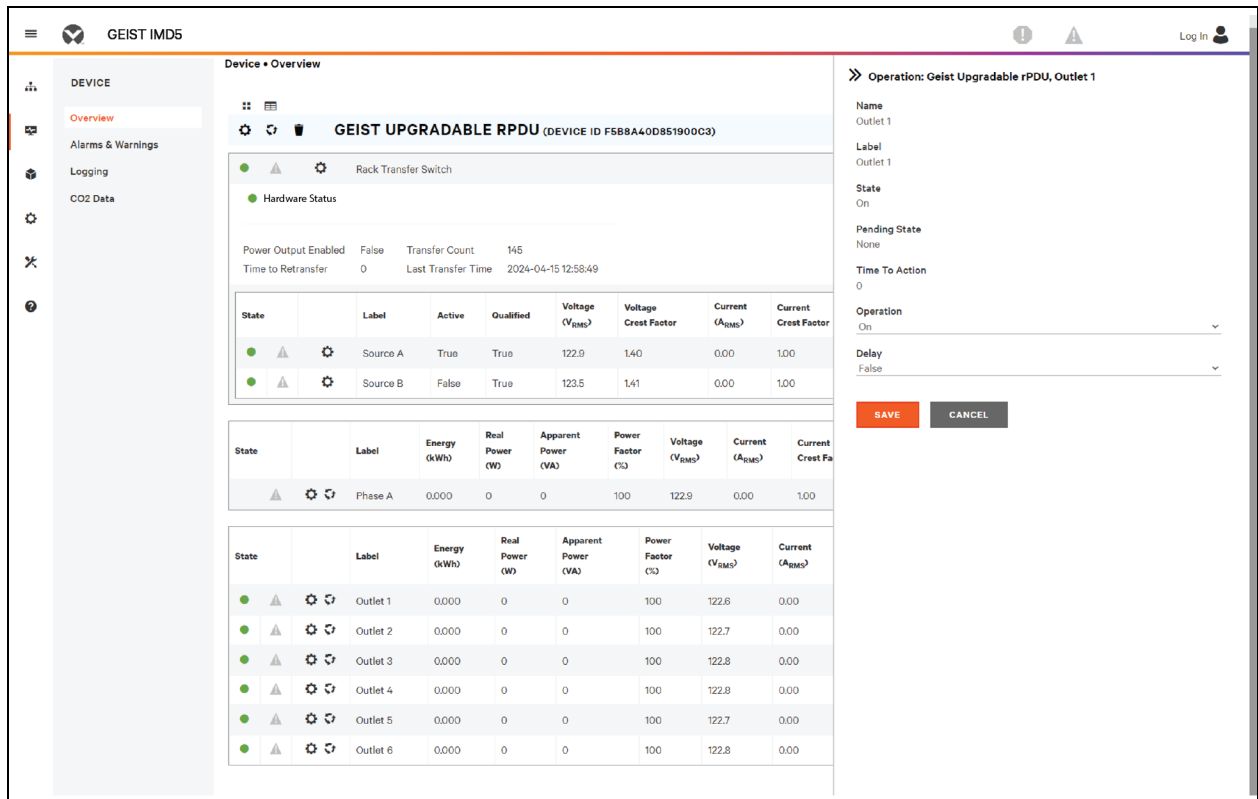
Figura 5.22 Cambio de la operación del tomacorriente
