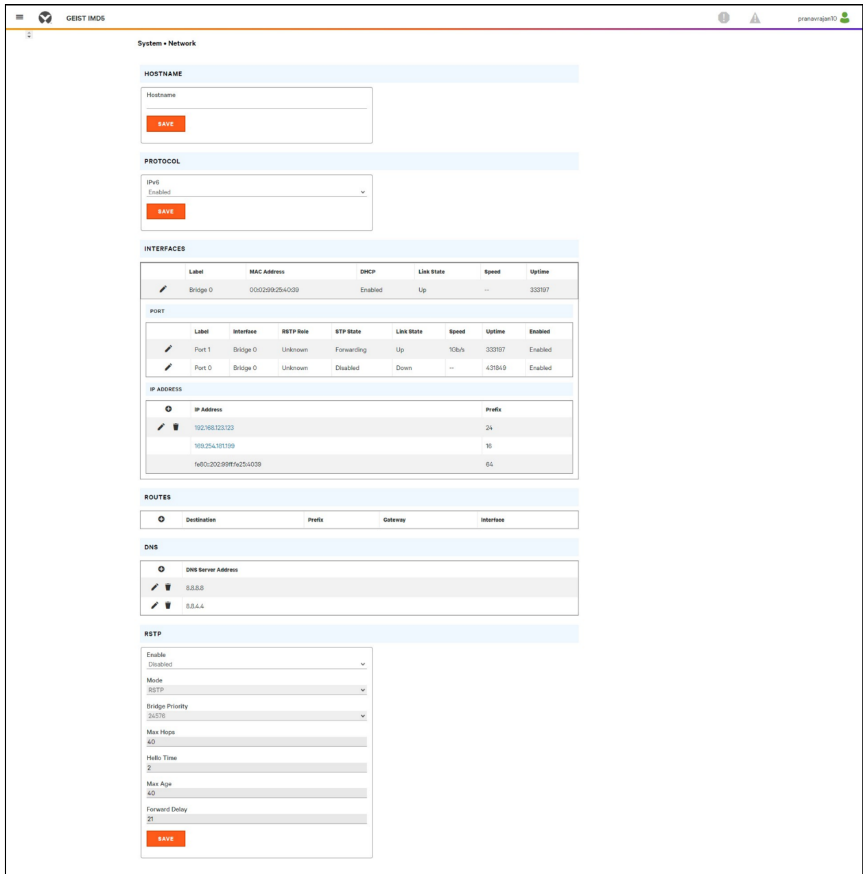
Figura 5.36 Página Network Configuration
