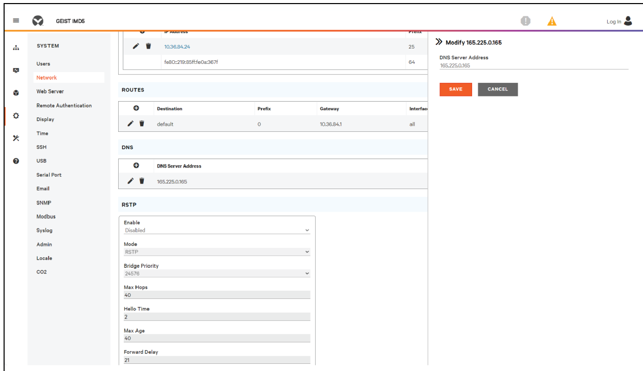
Figura 5.44 Modificar una dirección de servidor DNS
