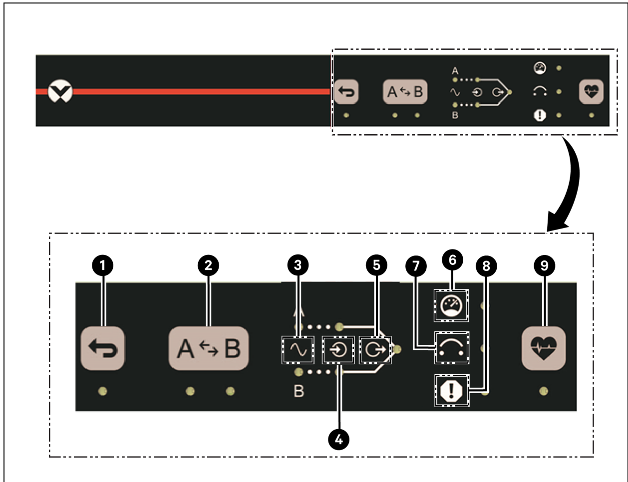
Figura 5.1 Visión general de la HMI
