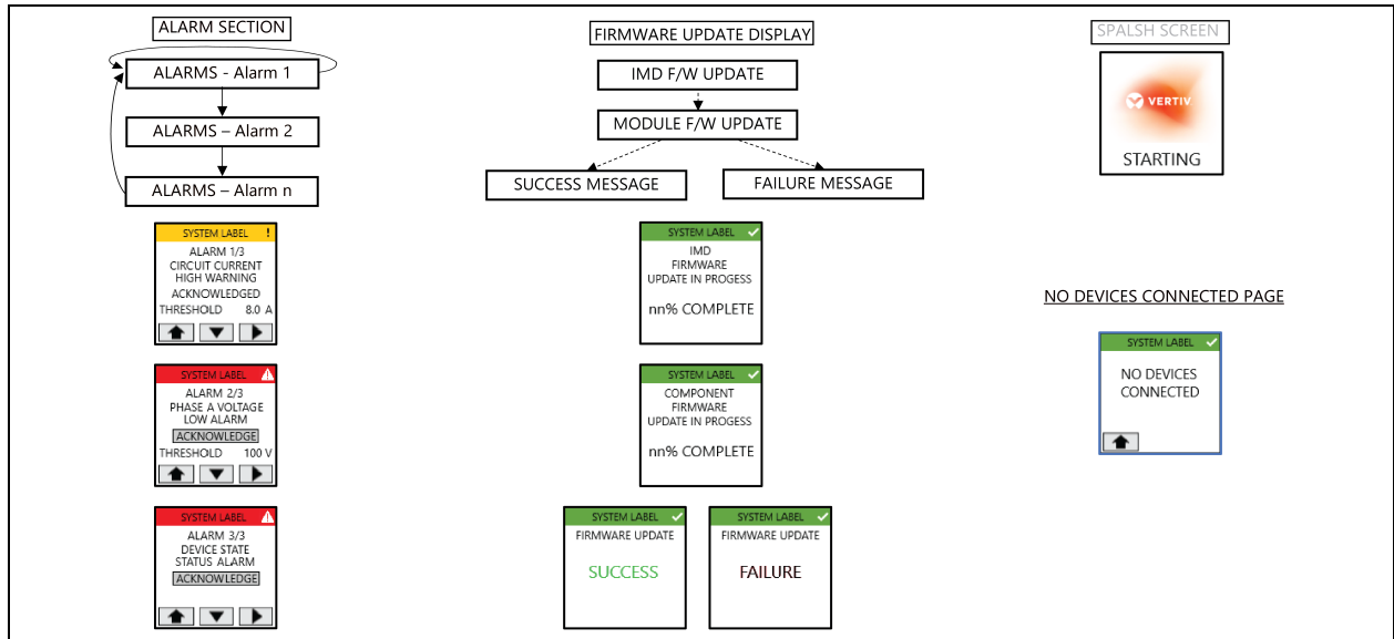
Figura 5.8 Sección de Alarm y Firmware Update Display
