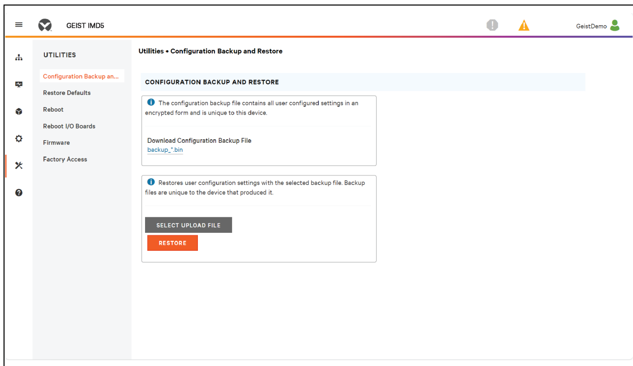
Figura 5.63 Información general de copia de seguridad y restauración de la configuración
