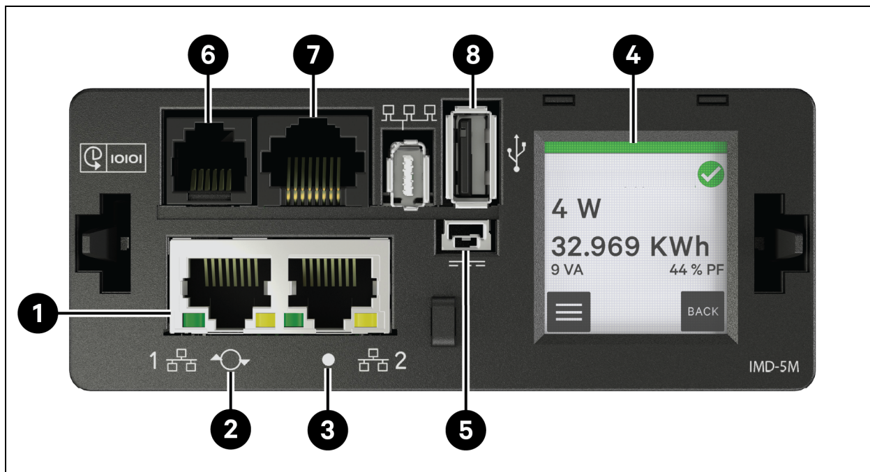
Abbildung 5.4 IMD-5M-Modul
