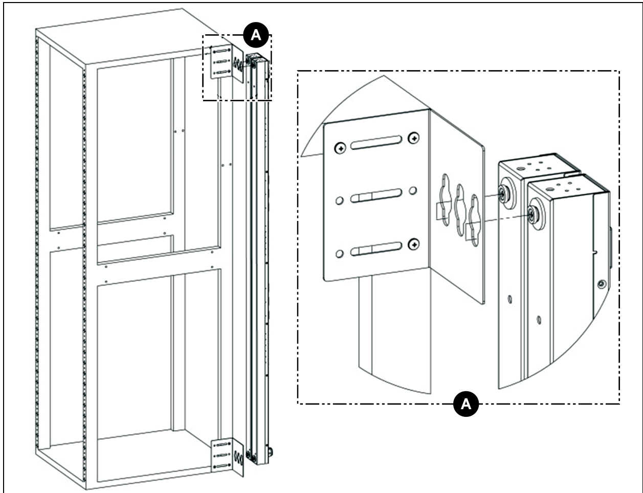
Abbildung 3.6 Halterungen zur einseitigen Montage für zwei Einheiten
