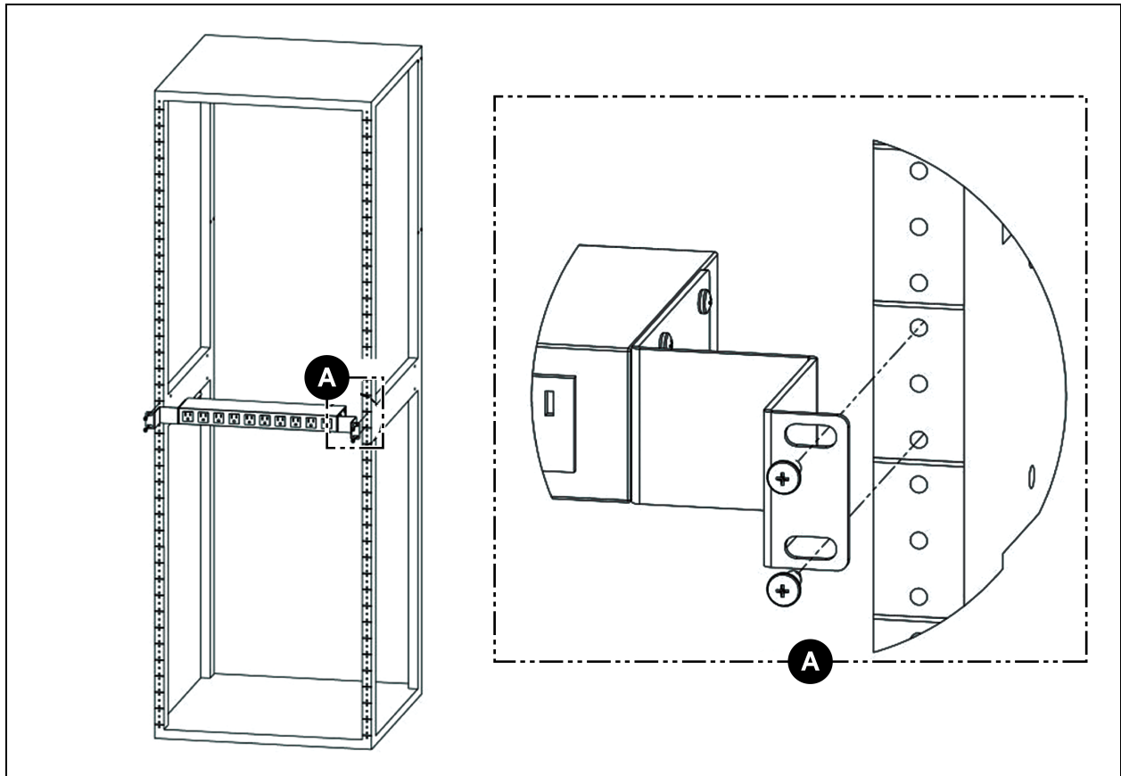
Abbildung 3.12 23-Zoll-Umrüstungs-Montagehalterungen
