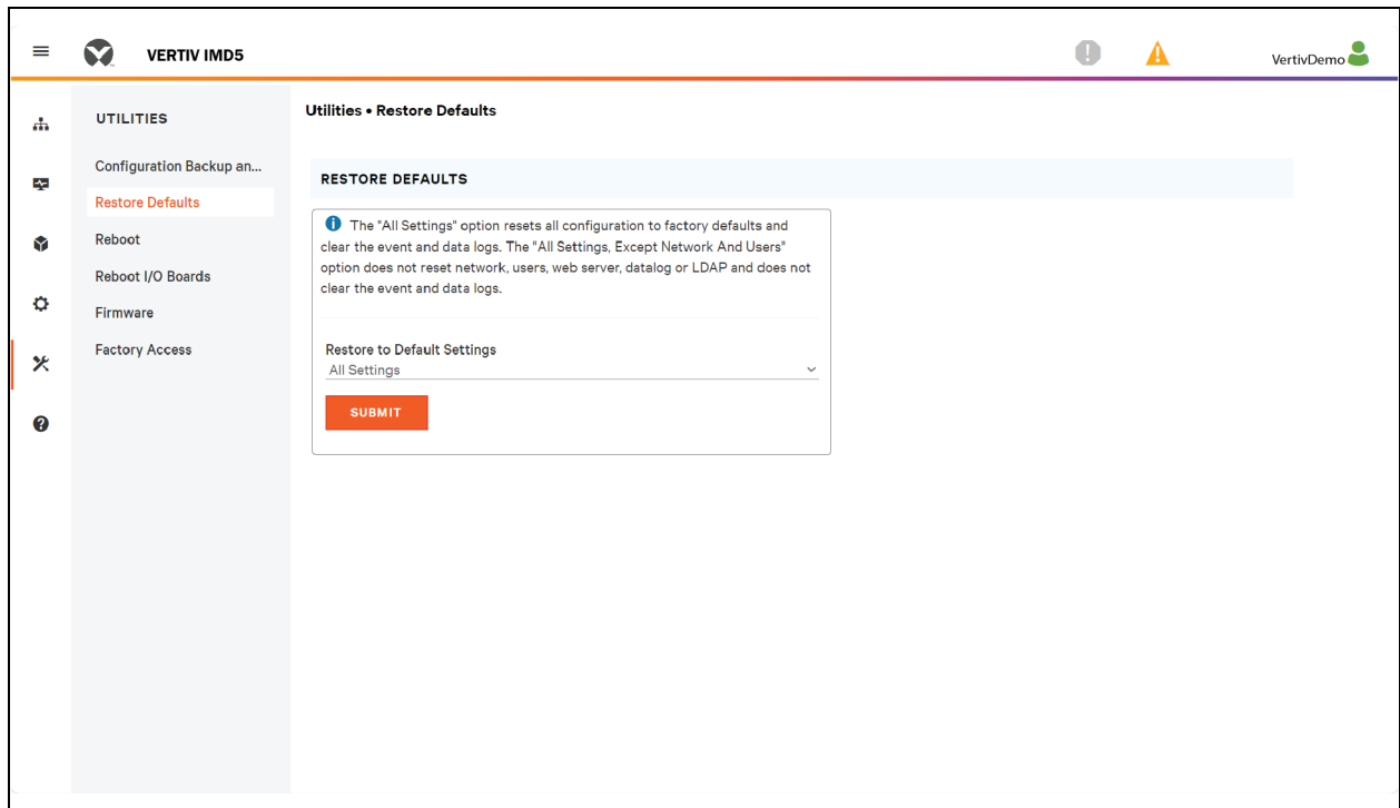
Abbildung 5.62 Überblick über Restore Defaults
