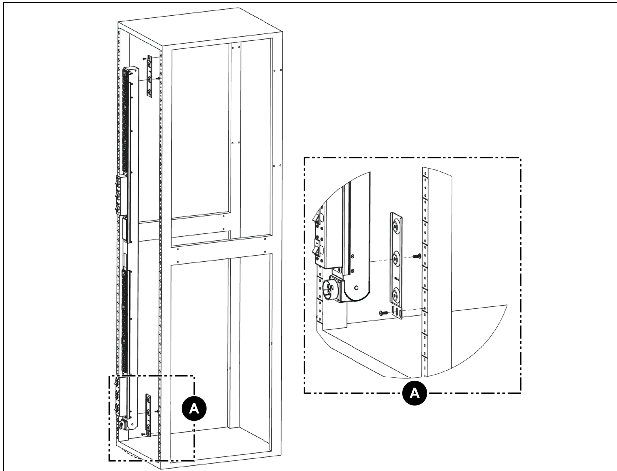
Abbildung 3.14 Montagehalterungen für Vertiv™ PowerIT Universal Power Distribution Unit (UPDU) mit Schwenkkopf
