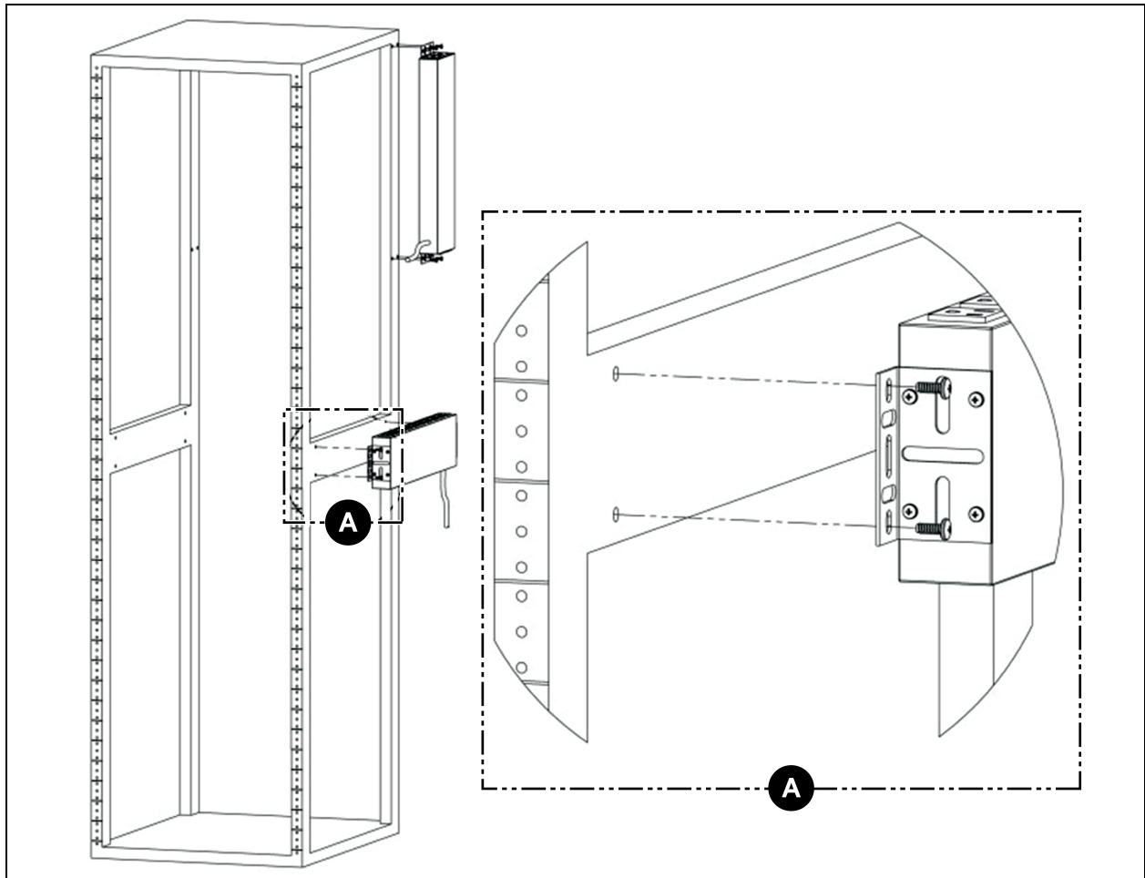
Abbildung 3.11 Panel-Montagehalterung
