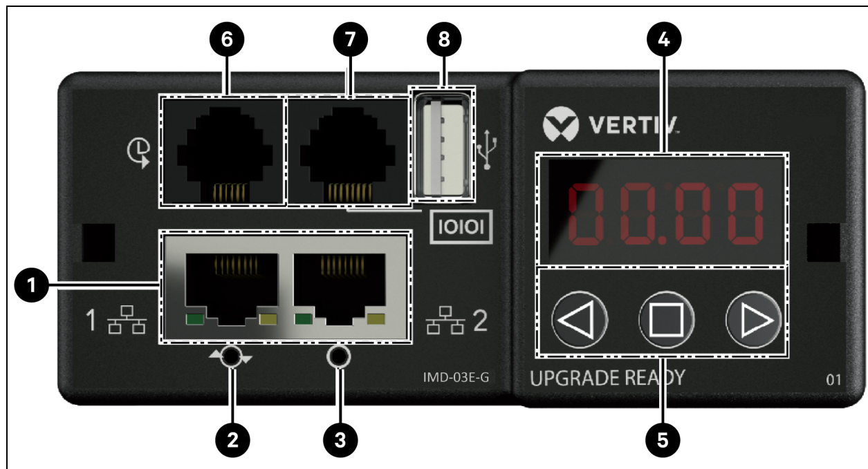
Abbildung 5.3 IMD-3E-G-Modul
