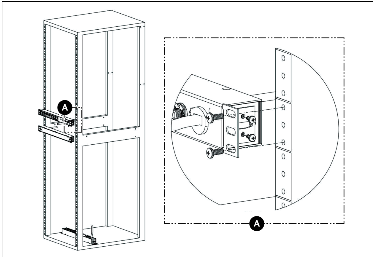
Abbildung 3.13 19 Zoll Horizontale/Panel-Montagehalterungen
