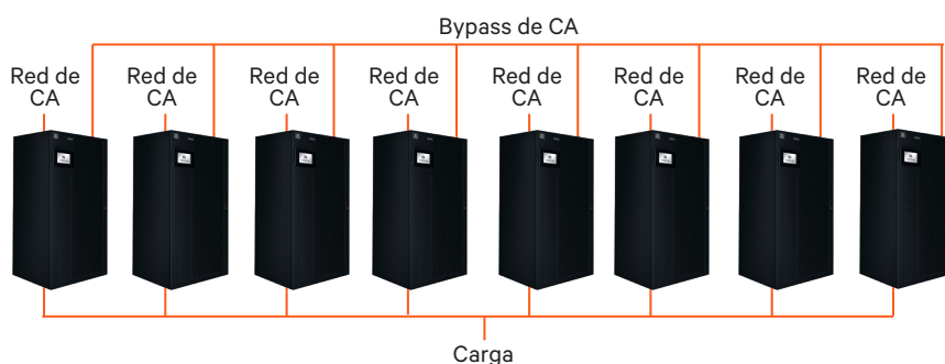
Configuración en paralelo distribuida de Vertiv™ Liebert® EXL S1, con 8 unidades UPS en paralelo
