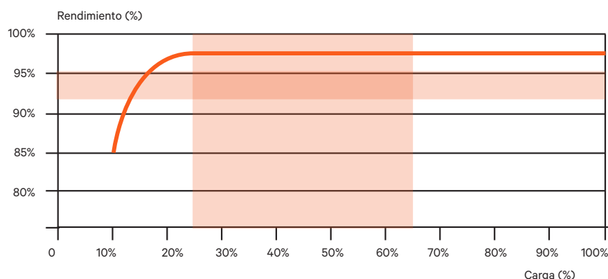
Rendimiento de CA/CA de Liebert EXL S1 con función de paralelo inteligente. Source: Vertiv Factory
