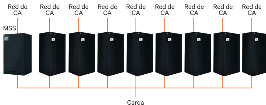
Configuración en paralelo centralizada de Vertiv™ Liebert® EXL S1, con MSS además de 8 unidades UPS en paralelo
