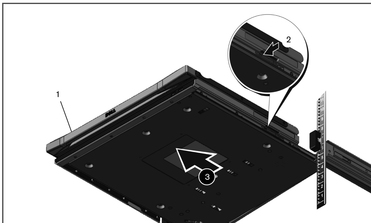
Рис. 4.1 Извлечение лотка консоли из стойки
