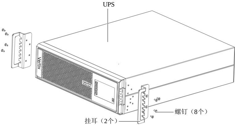
图2-10 安装挂耳
