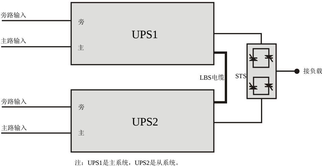
图3-8 LBS 系统示意图
