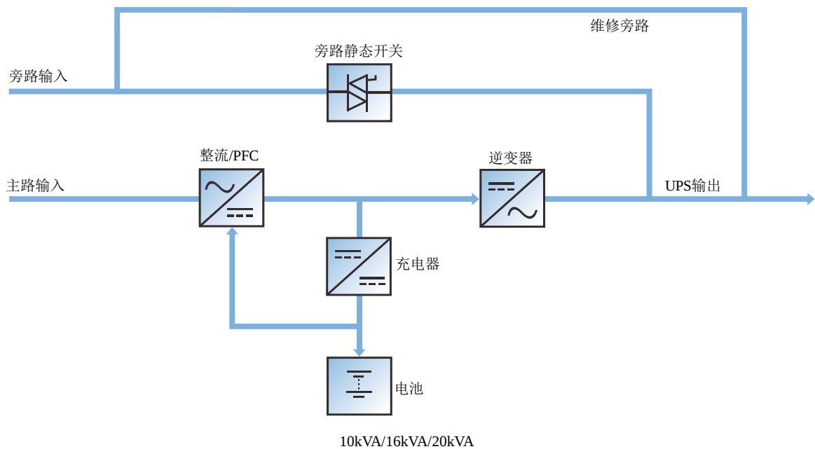
10kVA/16kVA/20kVA 图1-4 UPS 工作原理
