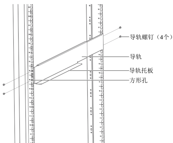
图2-13 安装导轨
