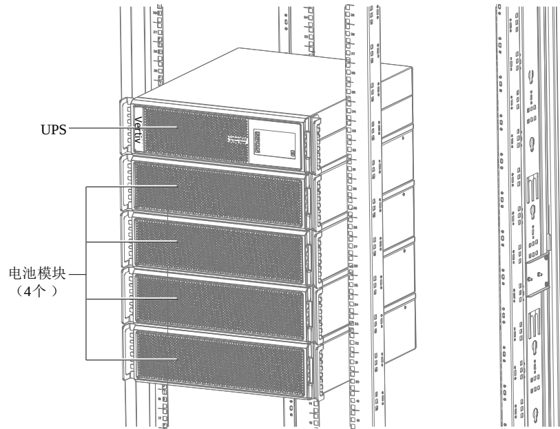
图2-16 带电池模块 UPS 安装示意图
