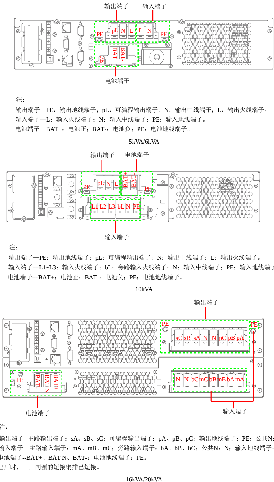
图2-17 输入输出端子排端子分布
