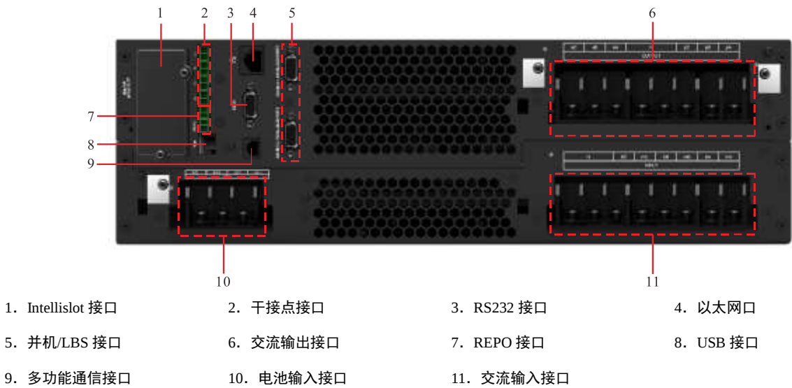
16kVA/20kVA 图1-3 UPS 后面板
