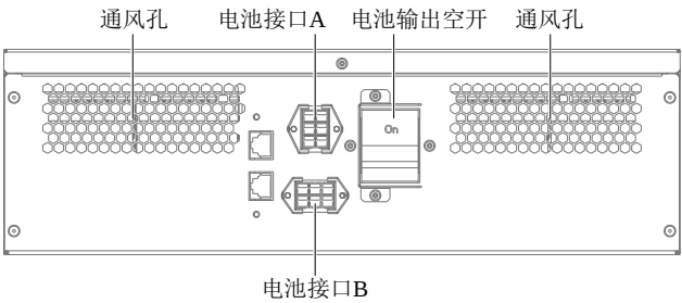
图8-3 电池模块后面板
