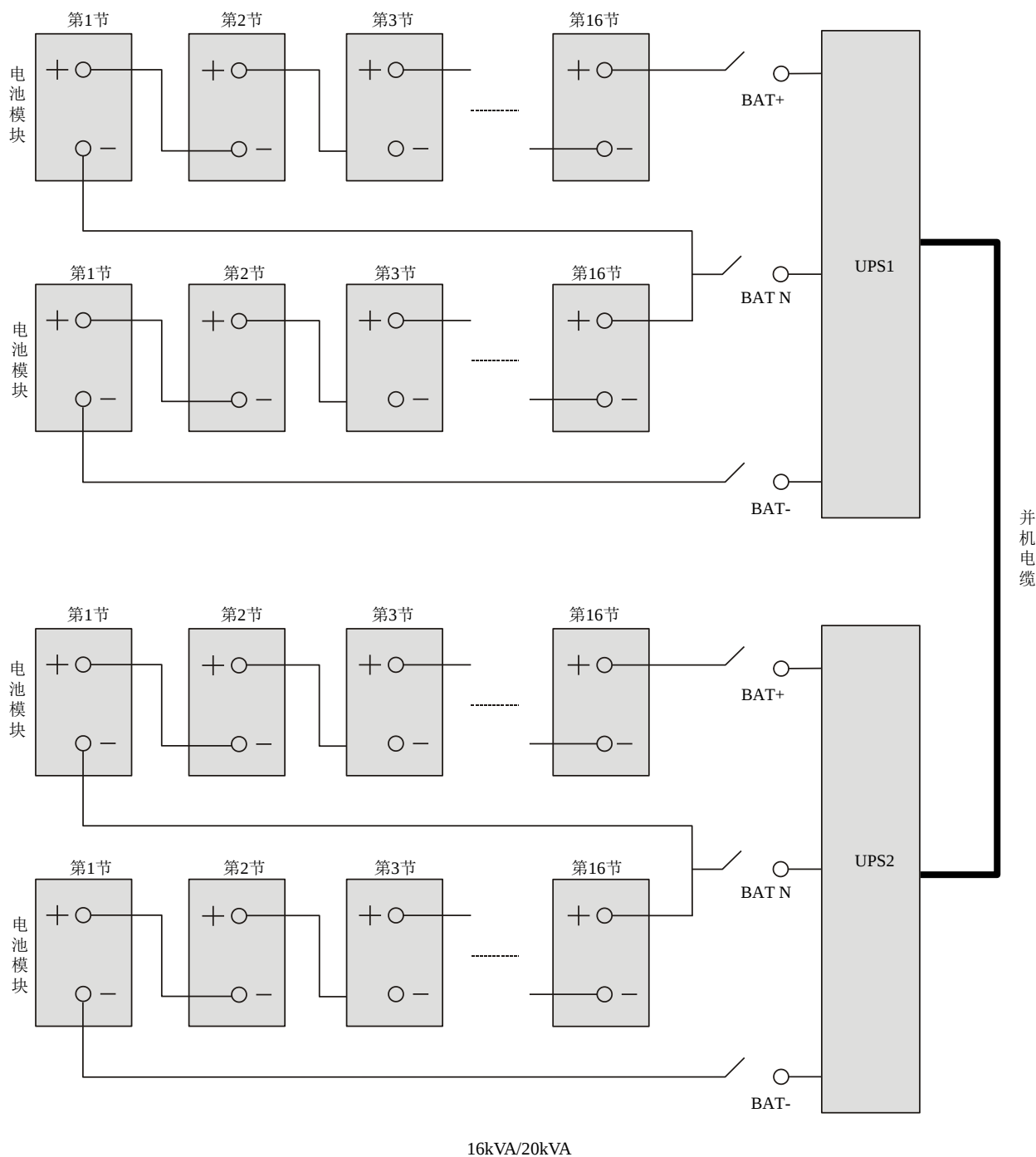
16kVA/20kVA 图3-4 独立使用电池组接线原理图
