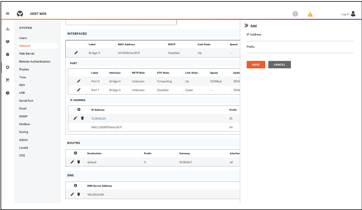
Figura 5.38 Adicionar um novo endereço IP
