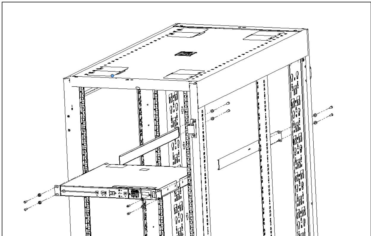
Figura 3.1 Suportes deslizantes do RTS
