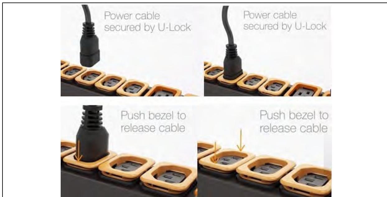
Figura 3.3 Operação de retenção de cabo U-Lock
