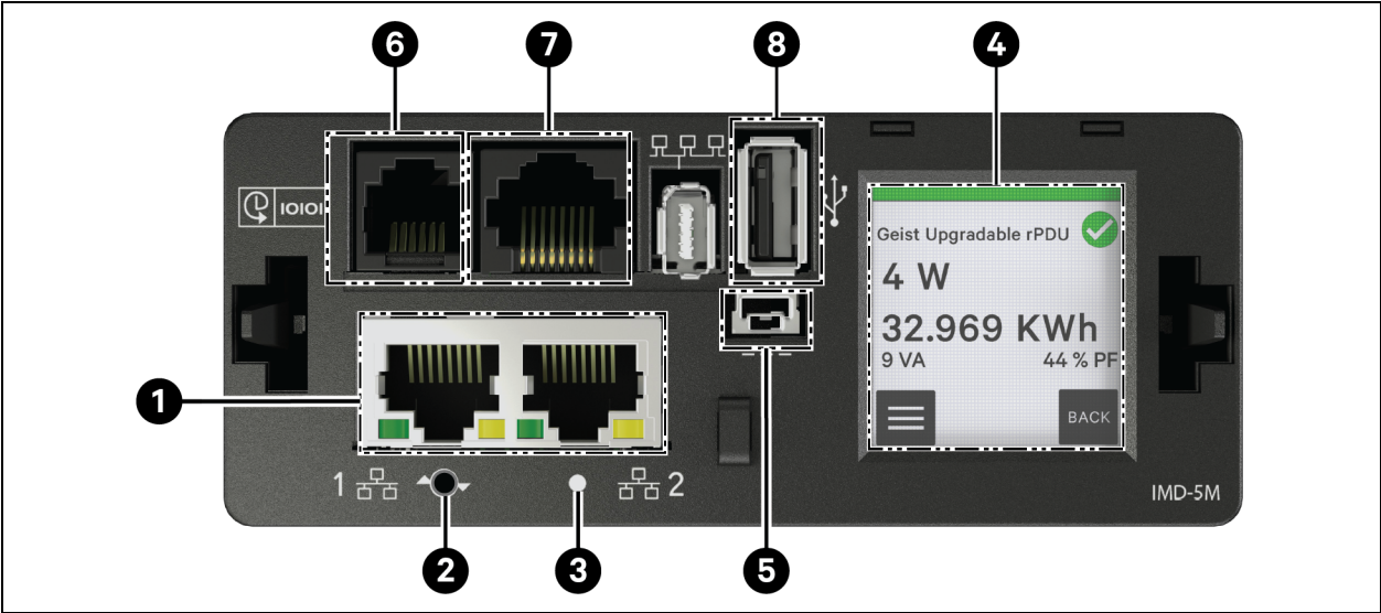
Figura 5.4 Módulo IMD-5M
