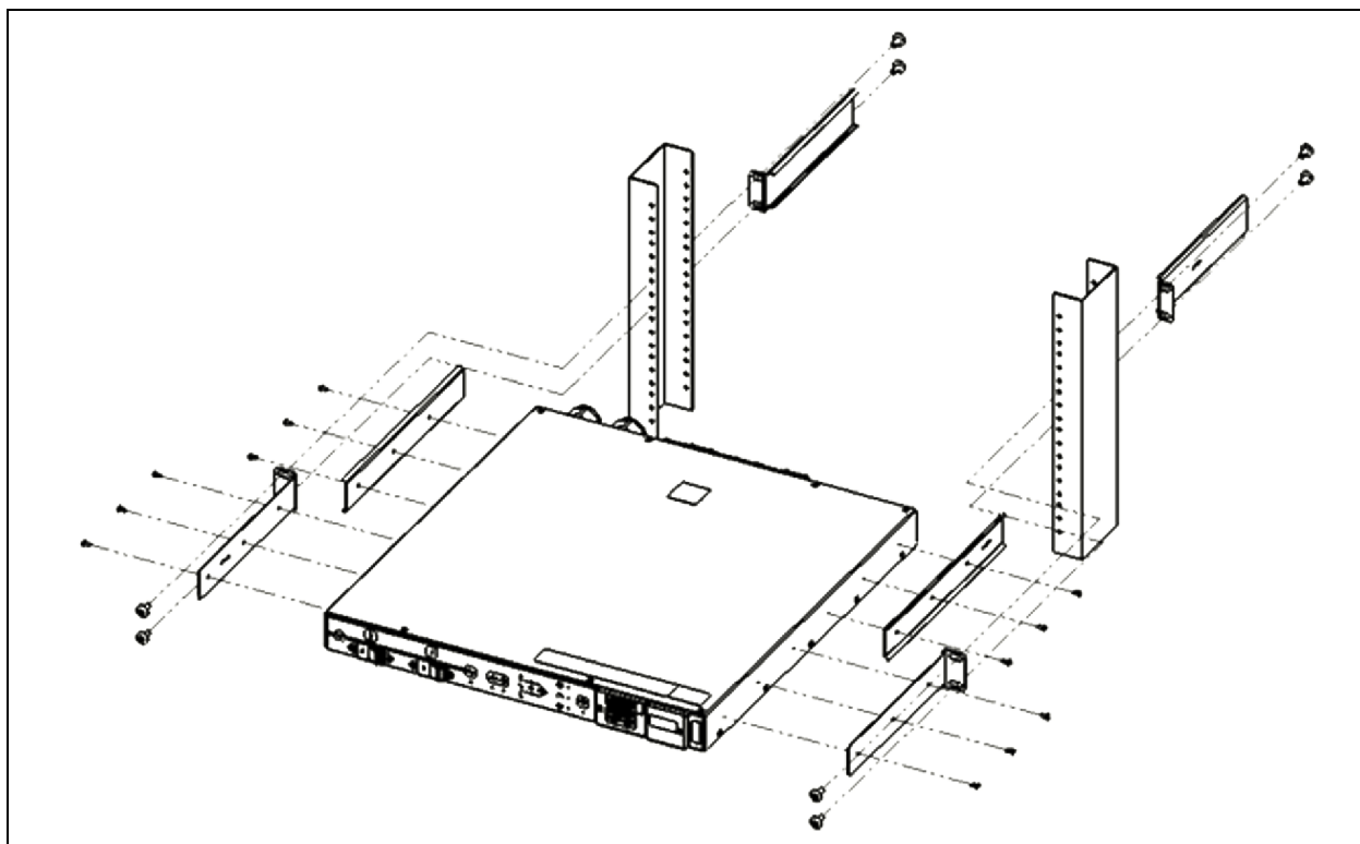
Figura 3.2 Suportes deslizantes do RTS
