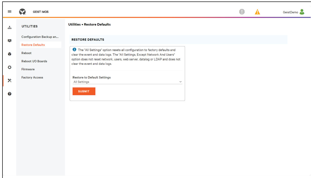
Figura 5.64 Visão geral de Restore Defaults
