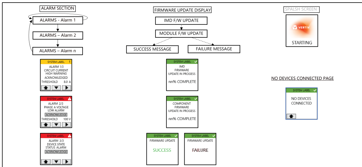
Figura 5.8 Seção Alarm e Exibição da atualização do firmware
