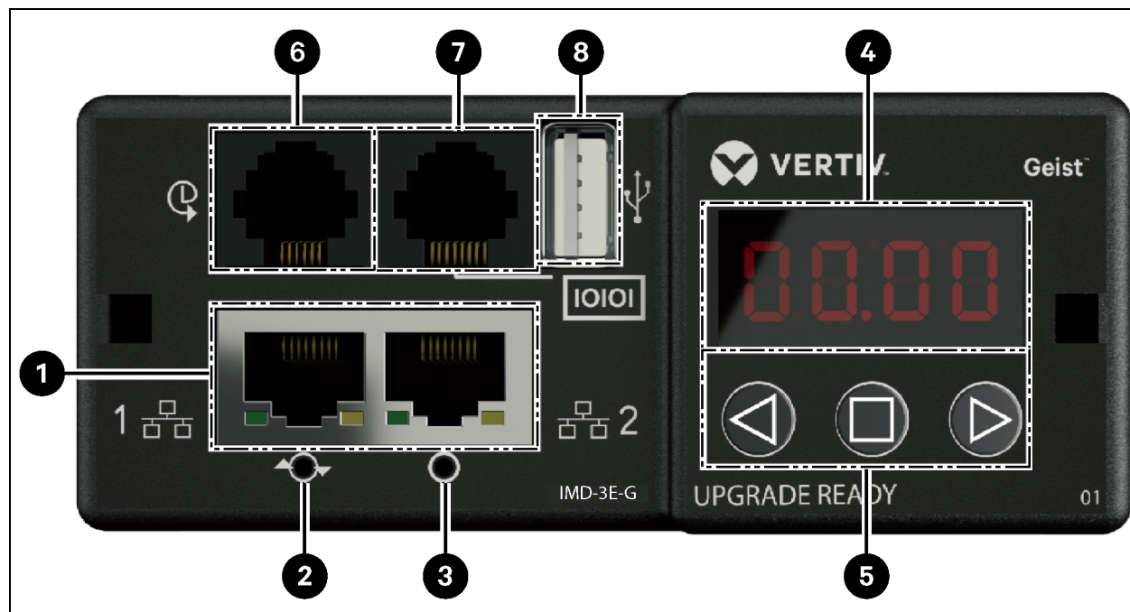
Figura 5.3 Módulo IMD-3E-G
