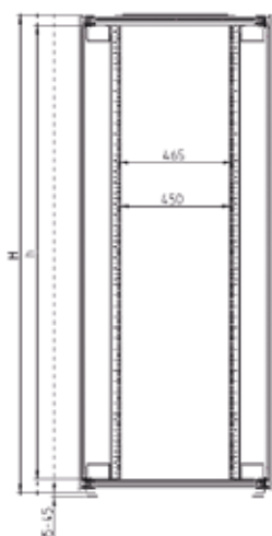
Rack serveurs Vertiv™ Knürr® MIR2
