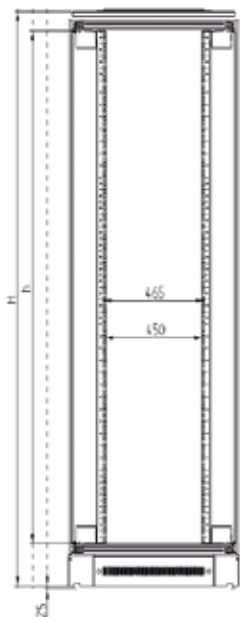
Rack réseau Vertiv™ Knürr® MIR2
